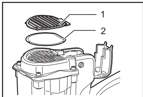
► 1. Couvercle du filtre 2. Filtre
